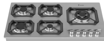
DS 523 سرشعله های SABAF راندمان بالا (HE) دارای شبکه چدنی لعاب کاری شده پنج تیکه Size: 890x510 mm Cut: 870x485 mm
